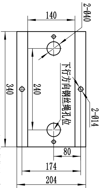
限速器安装位置示意图 请注意下行钢丝绳位置
