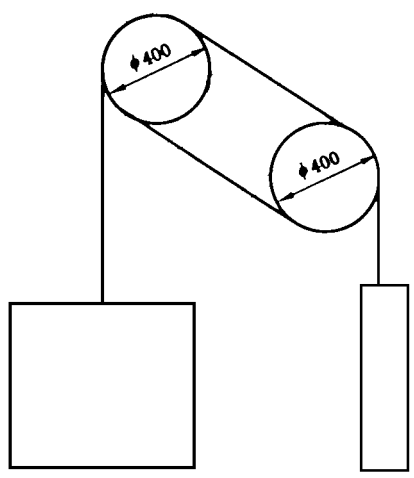
图 N2 滑轮等效数量的计算示例
