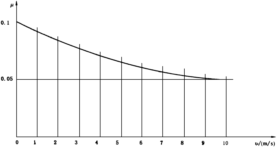
图 M3 最小的摩擦系数
