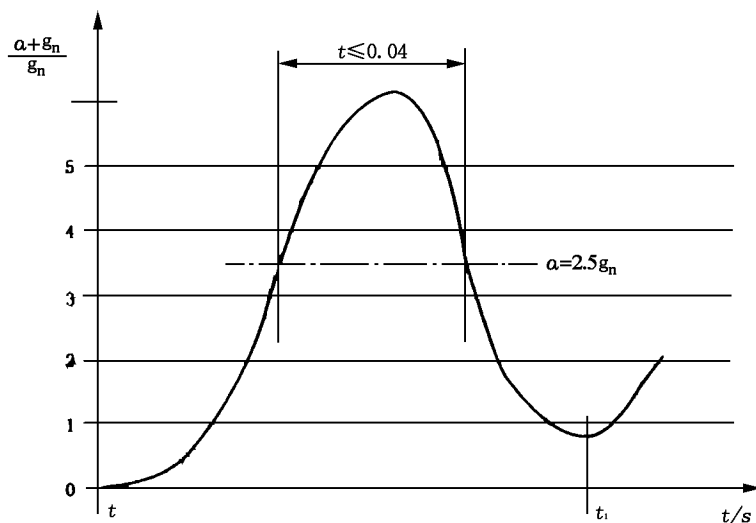
图 F1 减速度
