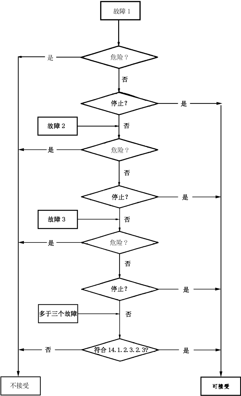
图 6 安全电路评价流程图
