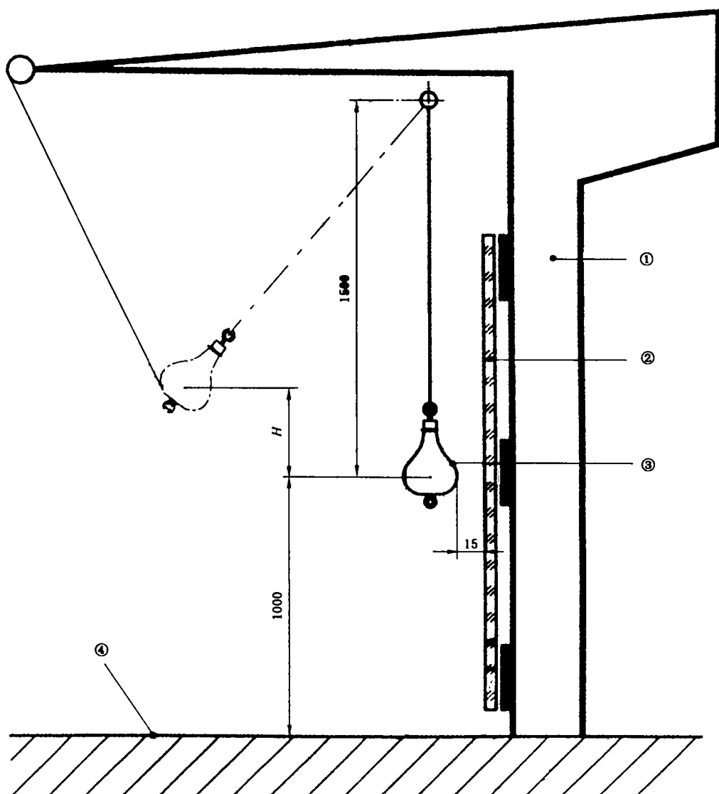
H —跌落高度；①—框架；②—被测试的玻璃面板； ③—冲击装置；④—被测试玻璃面板的参考地平面
