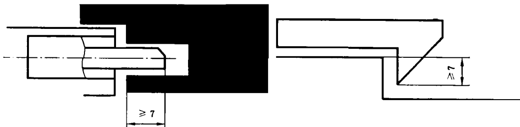
图 3 锁紧元件示例
