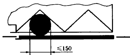
图 5 铰链层门和折叠轿门的间隙
