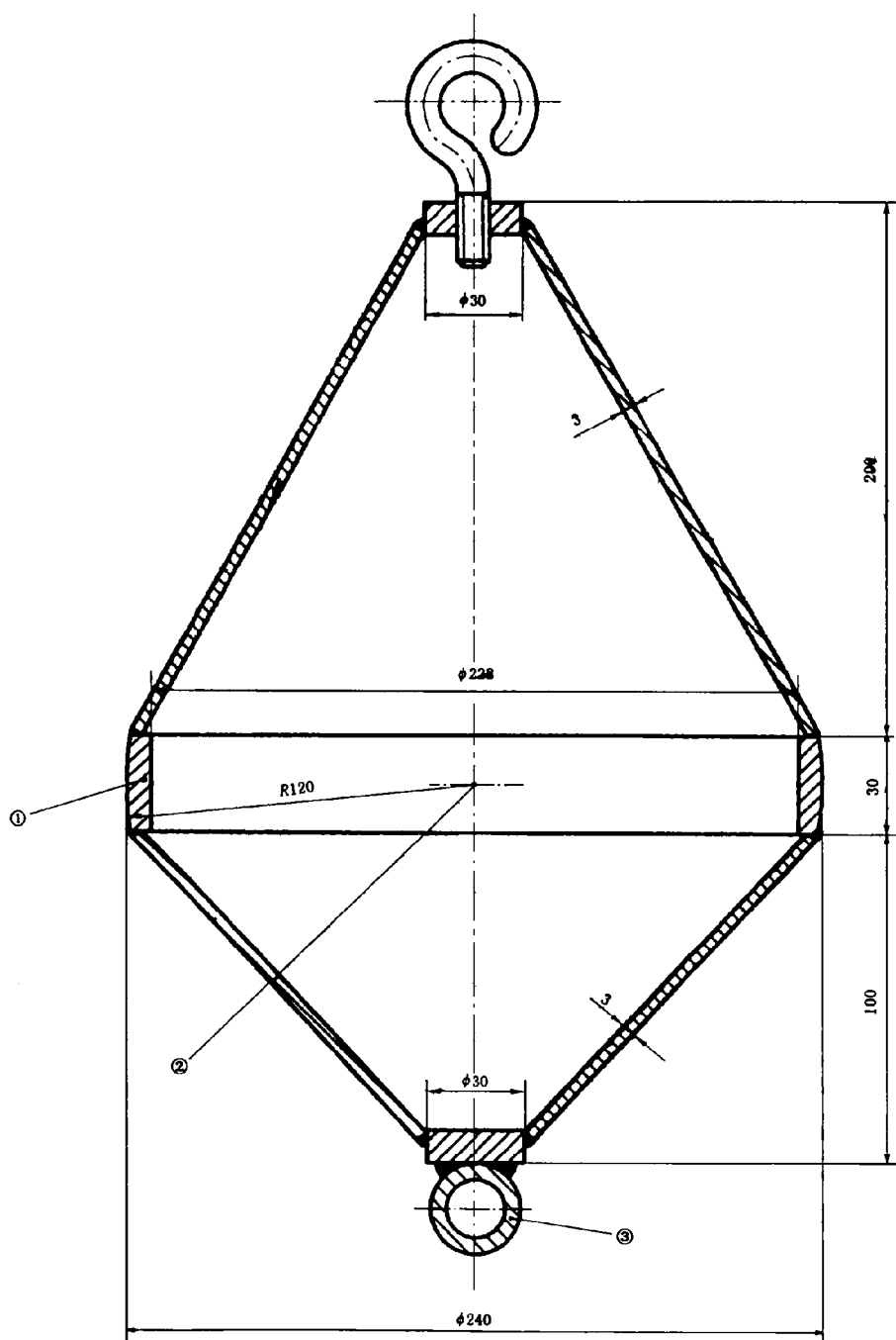
①—冲击环 ②—测量跌落高度参考点 ③—触发装置附件
