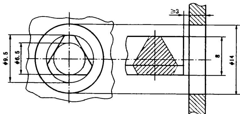
图 B1 开锁三角形钥匙
