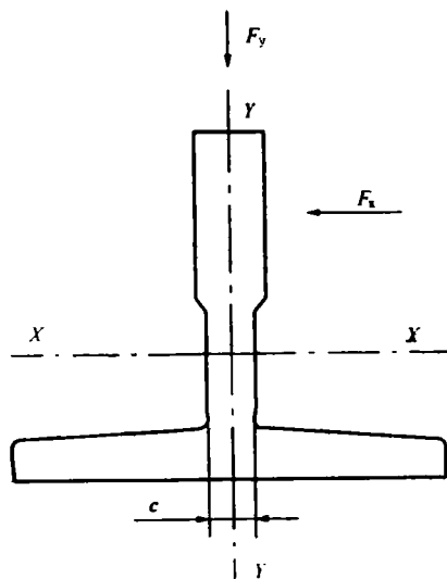
图 G1 导轨的坐标系
