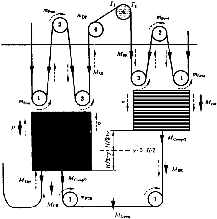
图 M4 通常情况
